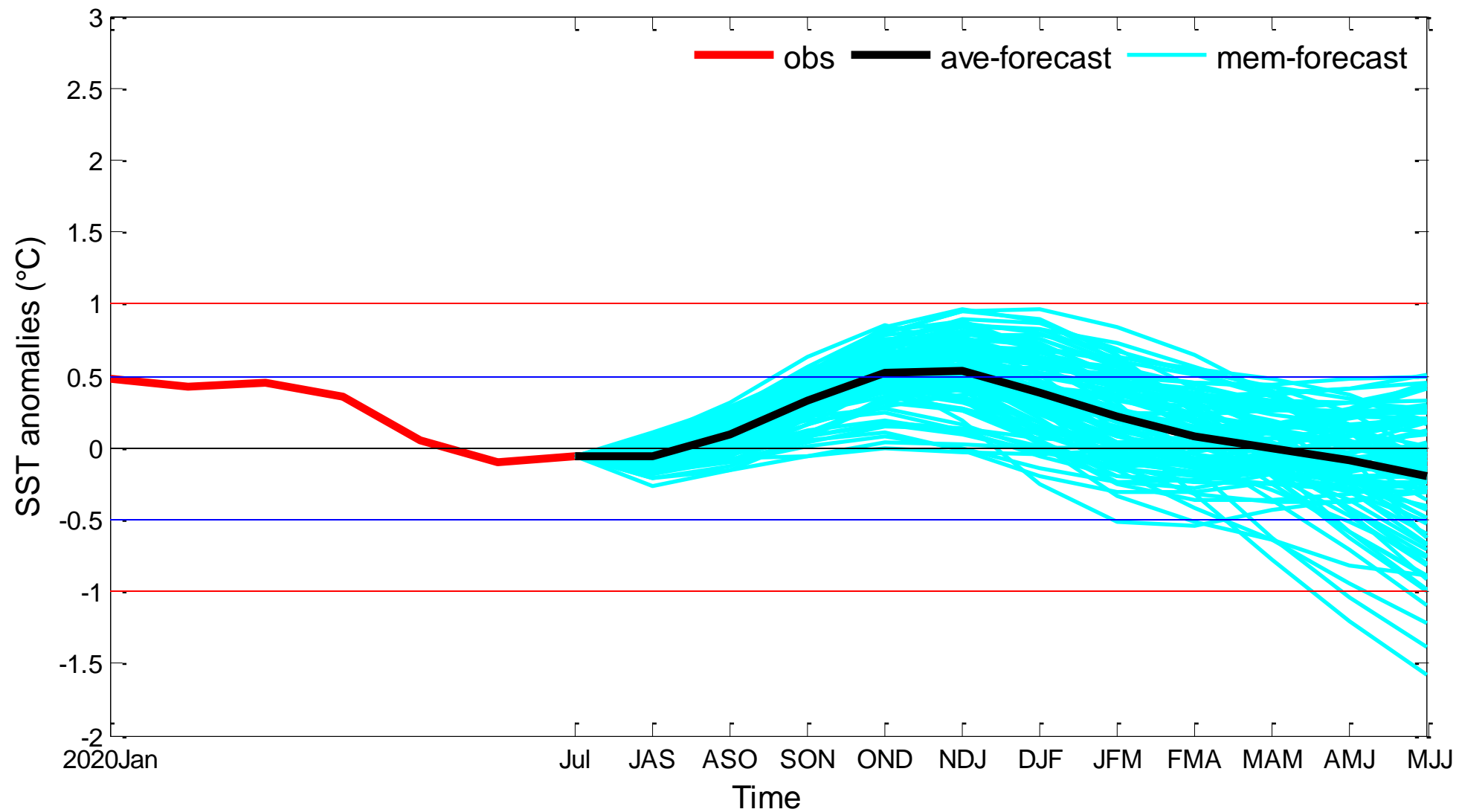
图1. Niño3.4指数的集合预报
