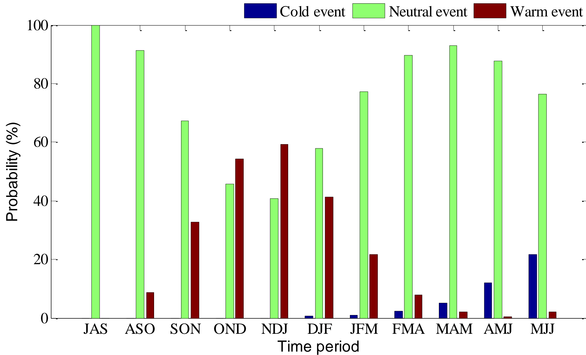
图2. 三类事件的概率预报
