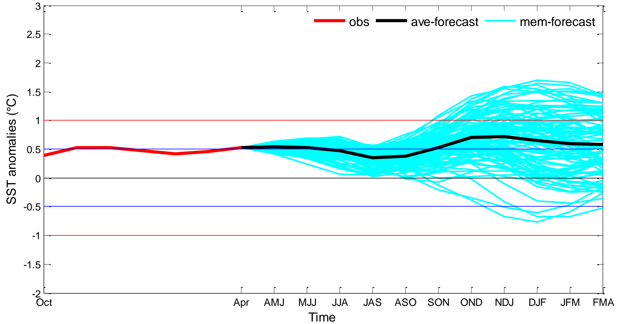
图1. Niño3.4指数的集合预报
