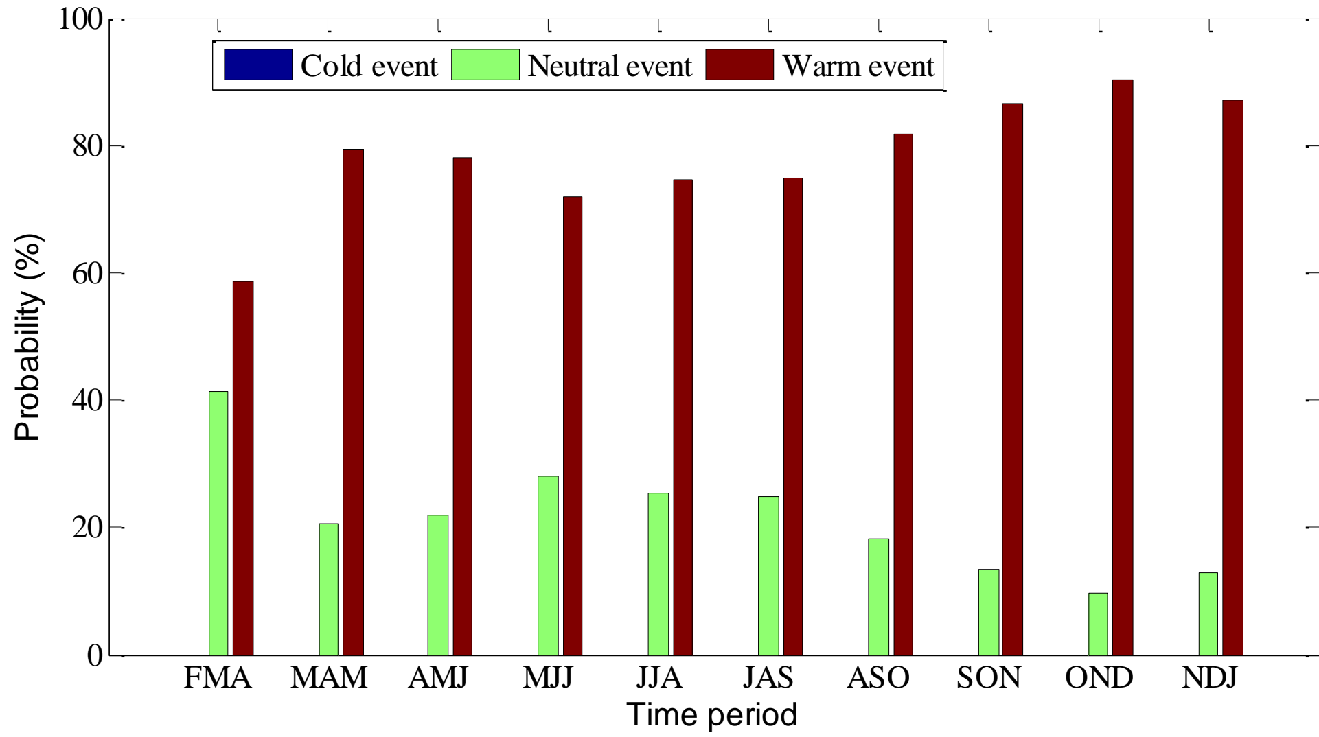
图2. 三类事件的概率预报
