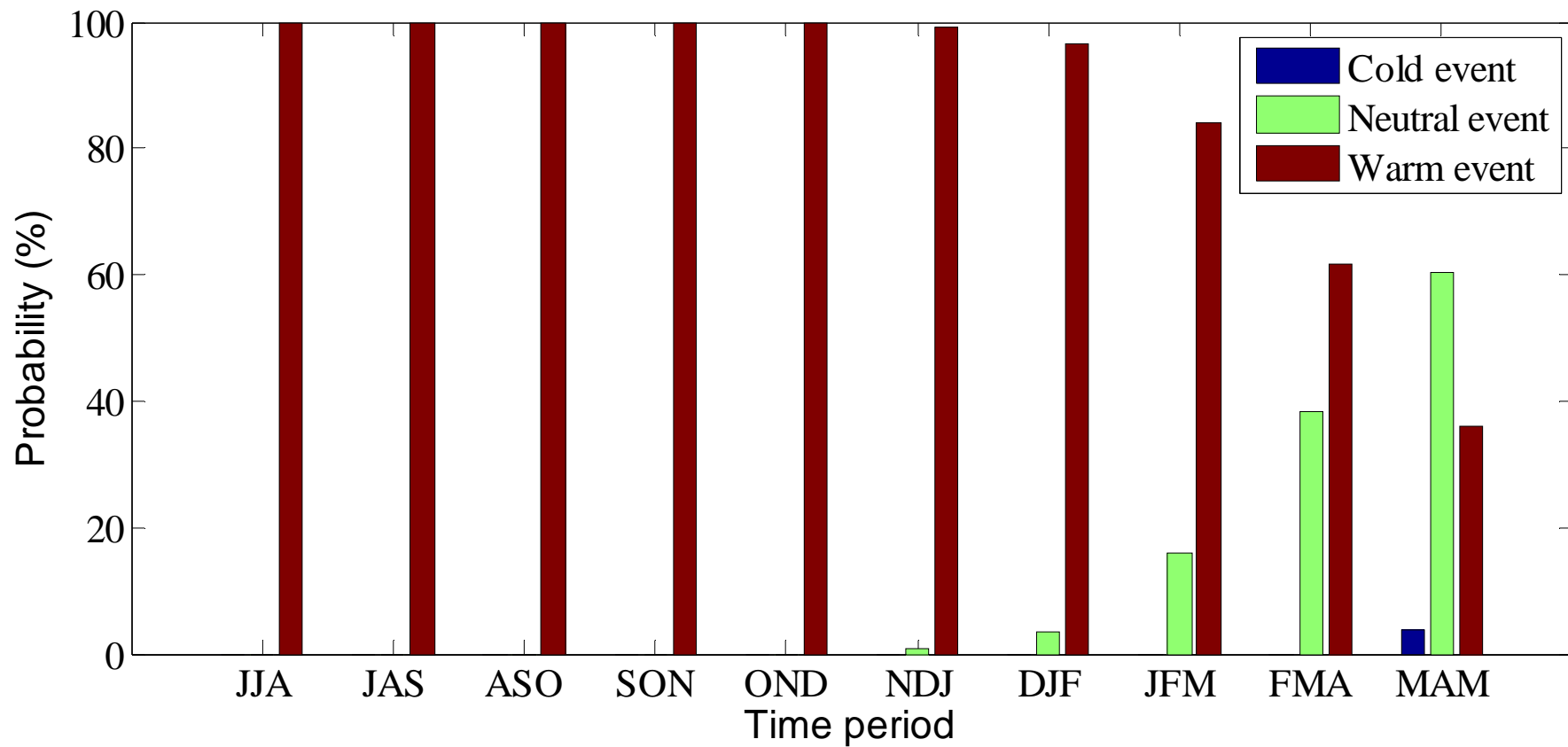
图2. 三类事件的概率预报
