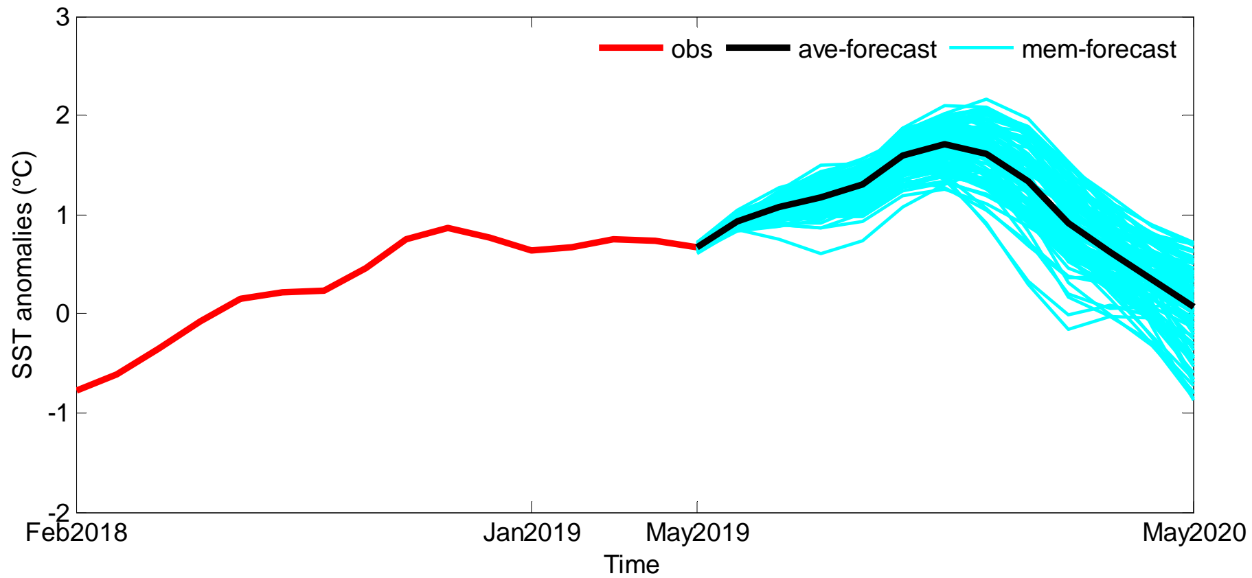
图1. Niño3.4指数的集合预报
