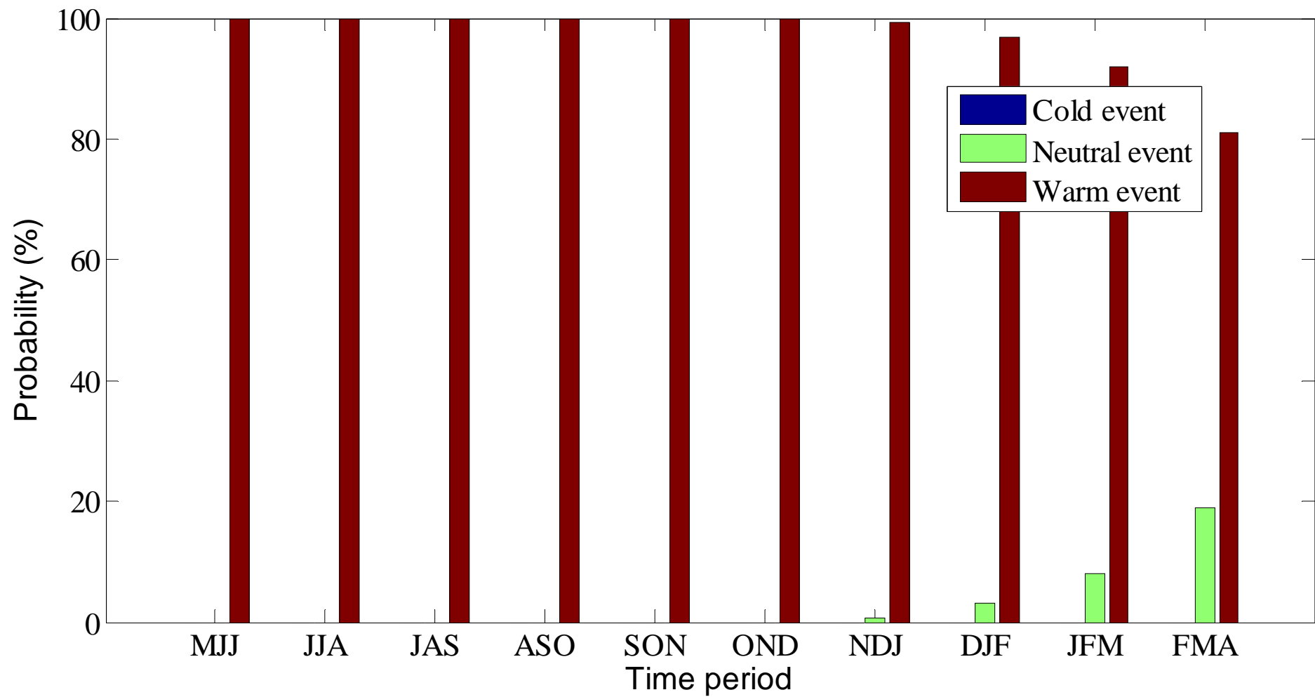
图2. 三类事件的概率预报
