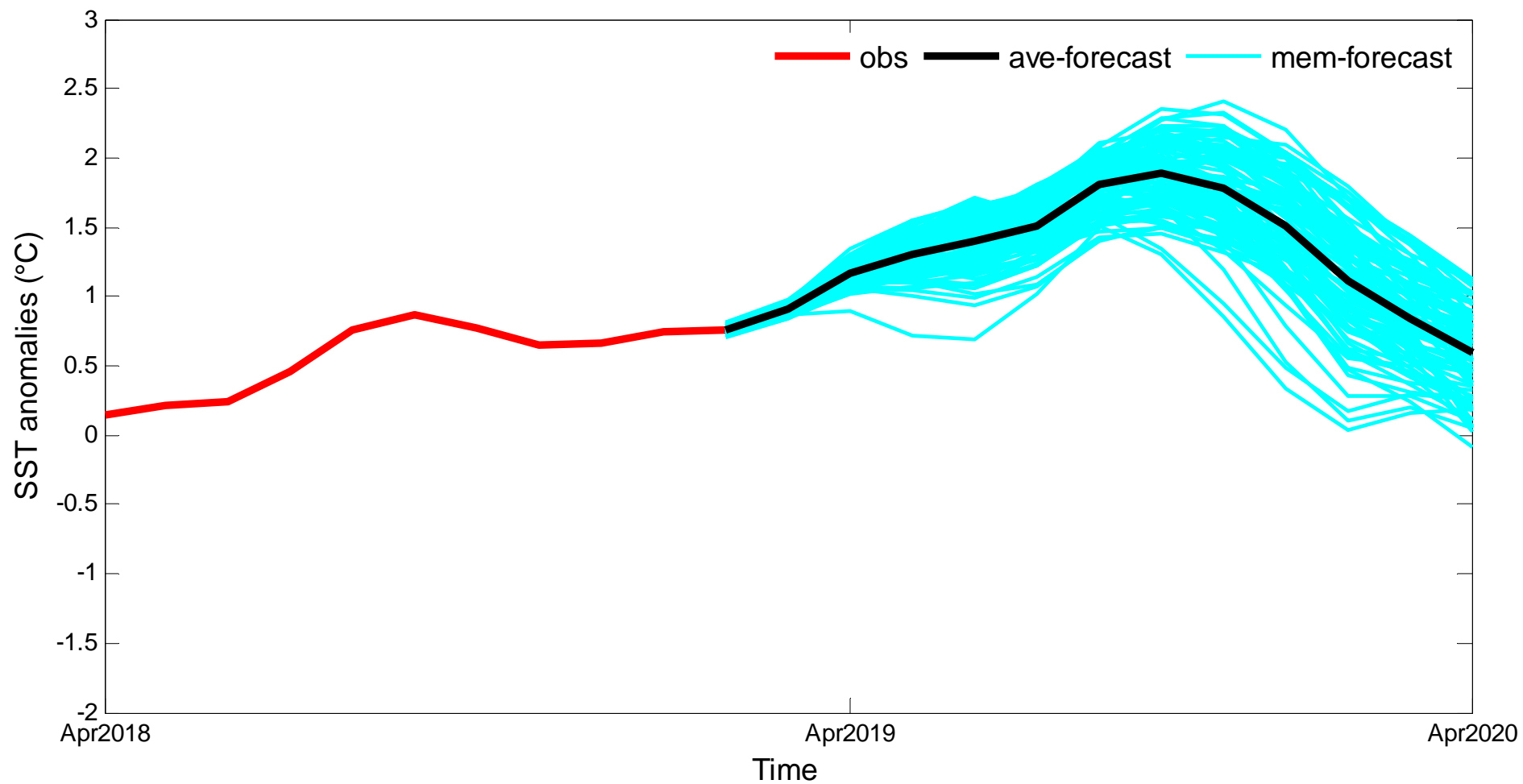
图1. Niño3.4指数的集合预报
