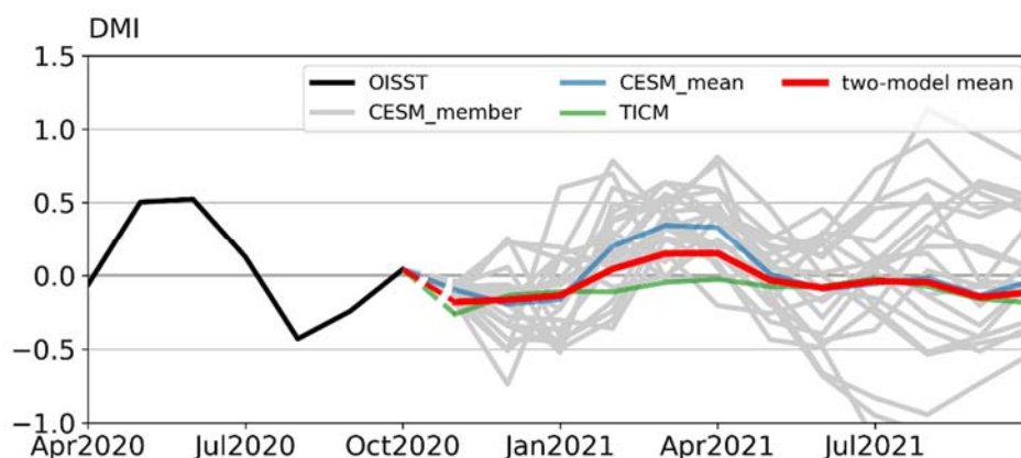
图 1 印度洋偶极子 (IOD) 实时预报系统于 2020 年 11 月起报 IOD 的确定性预报结果
