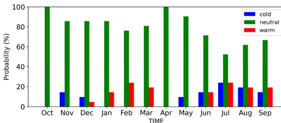
图 2 印度洋偶极子 (IOD) 实时预报系统于 2020 年 11 月起报 IOD 的概率预报结果
